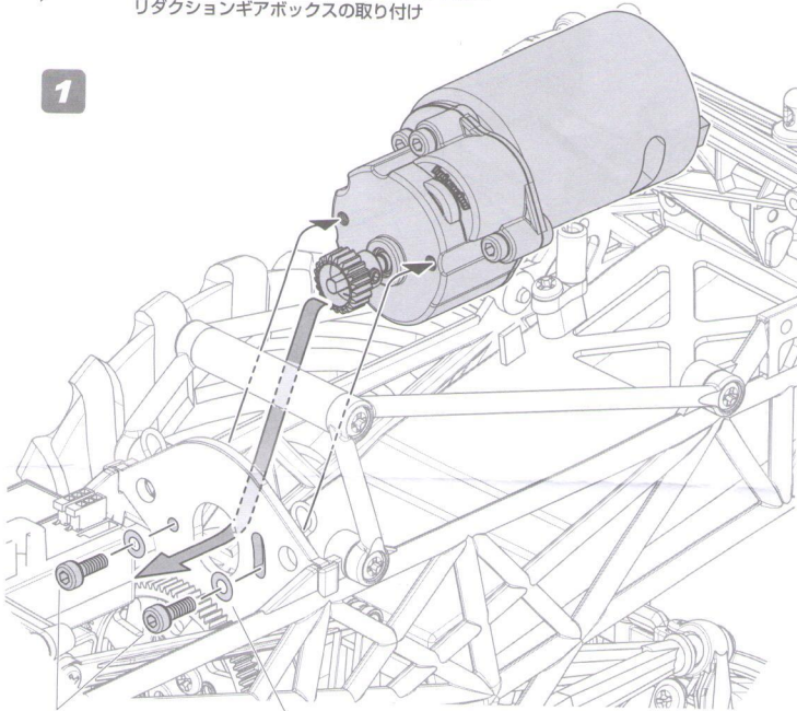
*Z541 Cap Head Screw M3x6mm Inbusschraube Vis tête cylindrique キャップスクリュー
